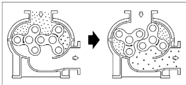
3葉形 ロータリーブロワの作動原理
